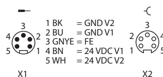
Abb. 19: TBEN-L5... – Pinbelegung Versorgungsspannungsanschlüsse
