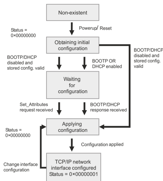
Abb. 55: TCP/IP Objektstatus-Diagramm (gemäß CIP Spez., Vol.2, Rev. 1.1)
