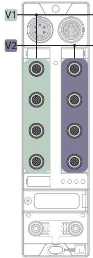
Abb. 20: Versorgung TBEN-L...-8IOL
