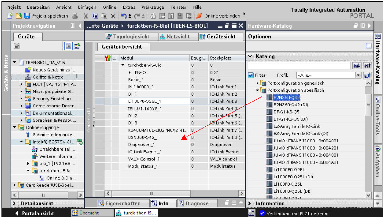
Abb. 43: TIA-Portal – Steckplätze des Geräts konfigurieren
