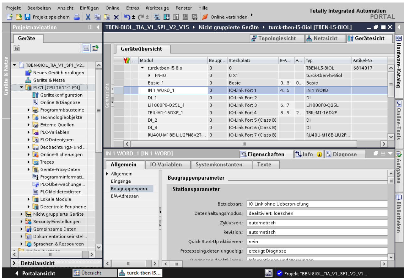
Abb. 44: TIA-Portal – Parametrieren generischer IO-Link-Devices
