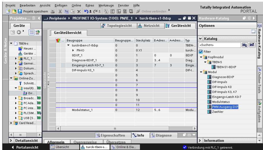
Abb. 36: TIA-Portal – Belegung der Slots und Subslots am Beispiel eines TBEN-S1-8DXP
