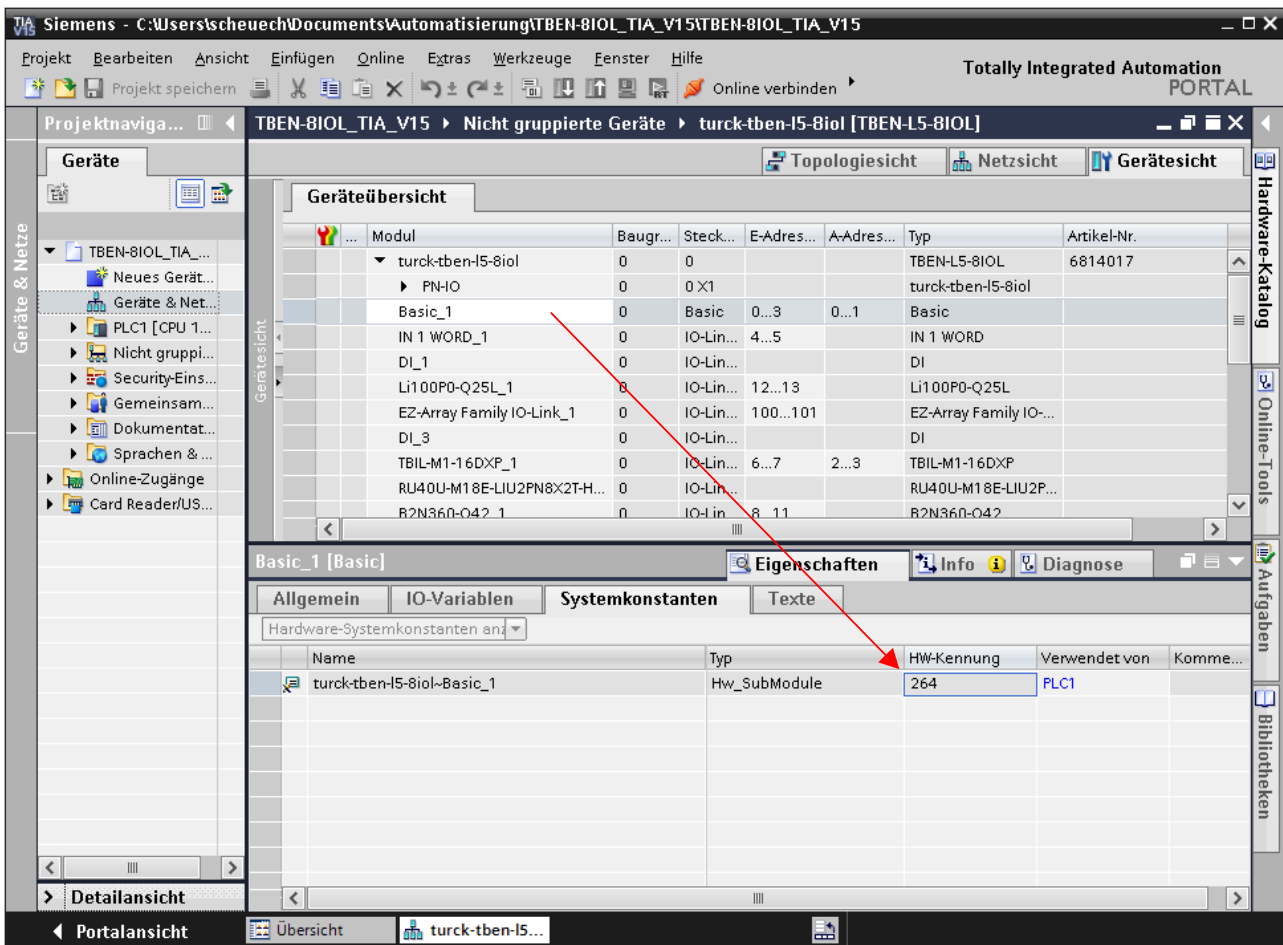
Abb. 47: HW-Kennung: „Basic“-Steckplatz des TBEN-L...-8IOL
