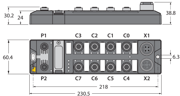
Abb. 4: Abmessungen TBEN-L4-8IOL
