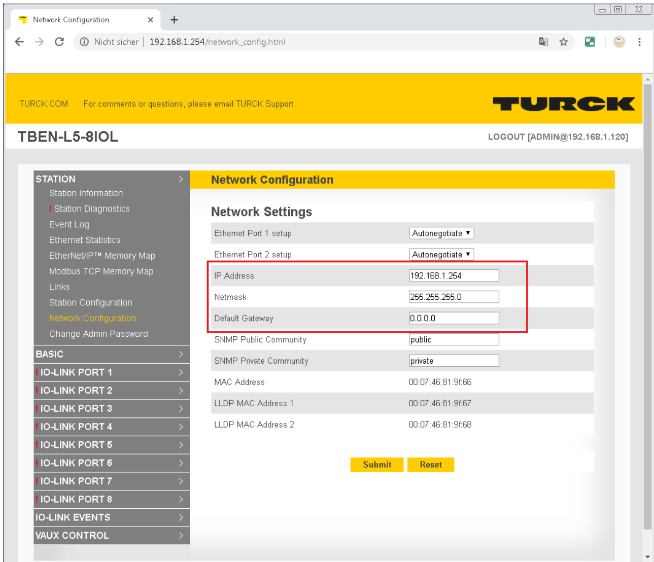
Abb. 30: IP-Adresse über den Webserver einstellen
