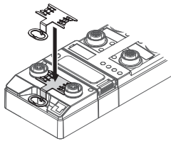
Abb. 13: Erdungsspanne montieren
