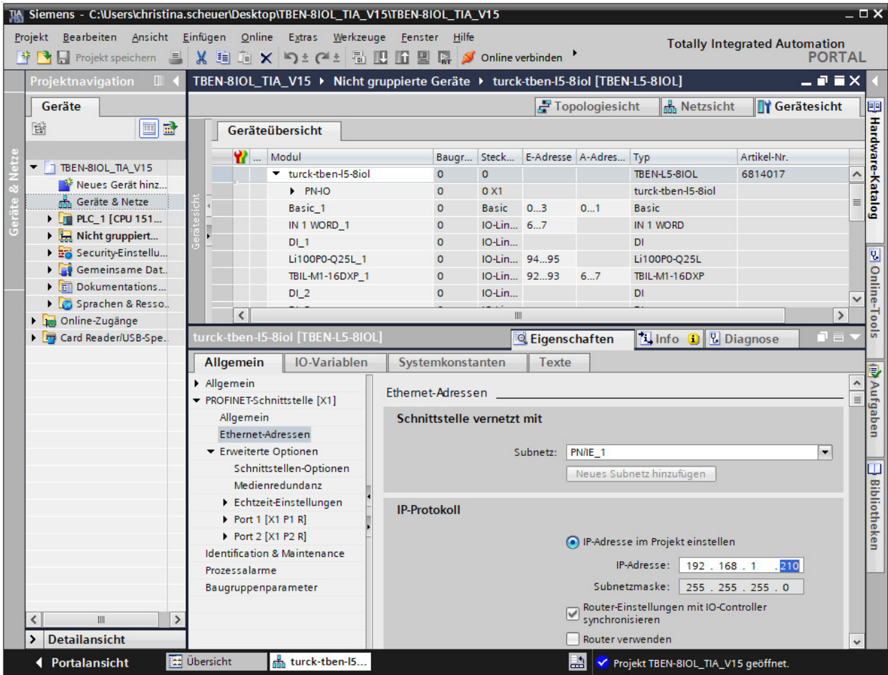
Abb. 42: IP-Adresse vergeben
