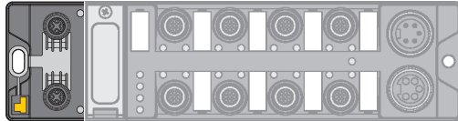
Abb. 14: M12-Ethernet-Steckverbinder
