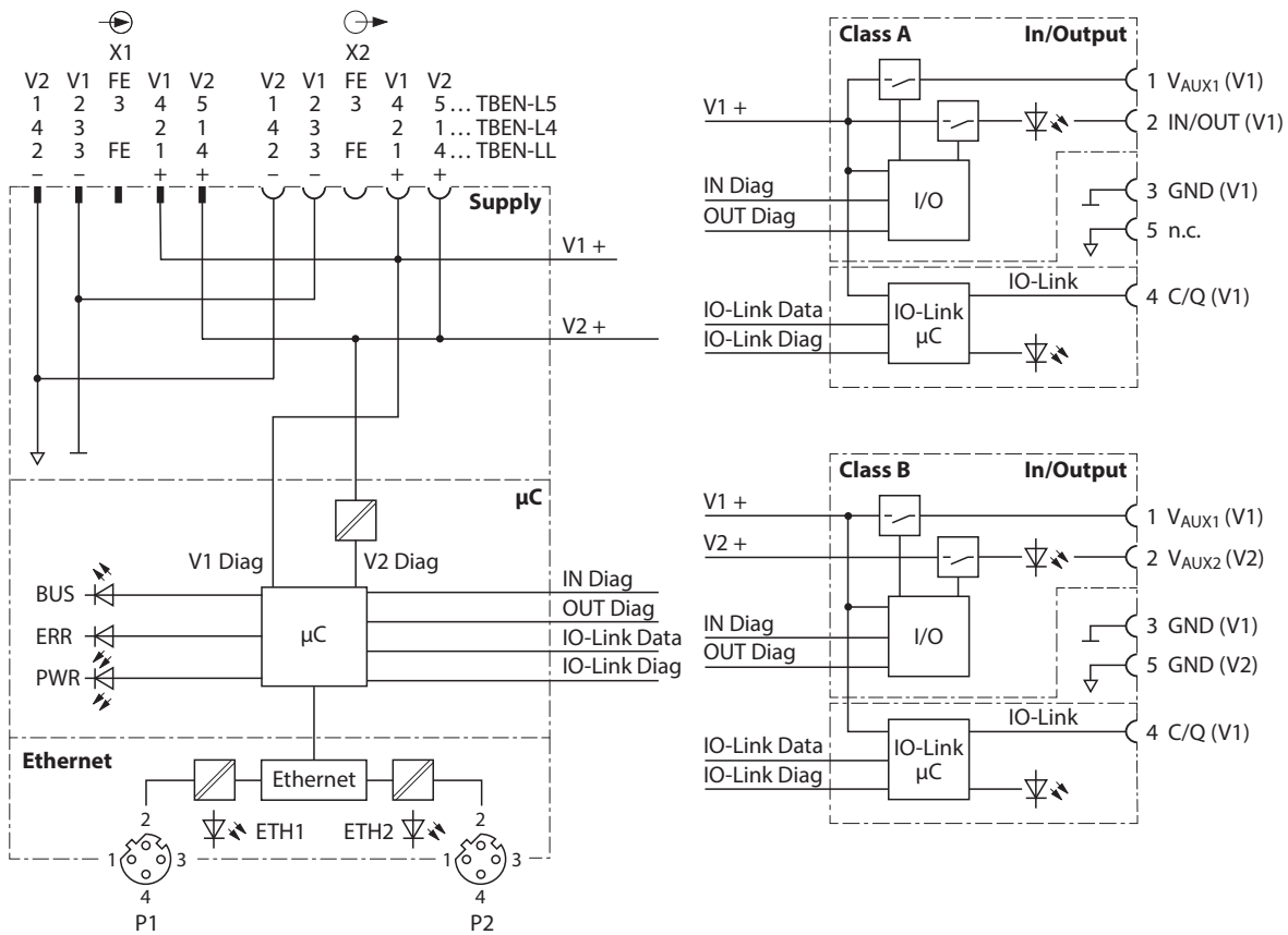
Abb. 6: Blockschaltbild
