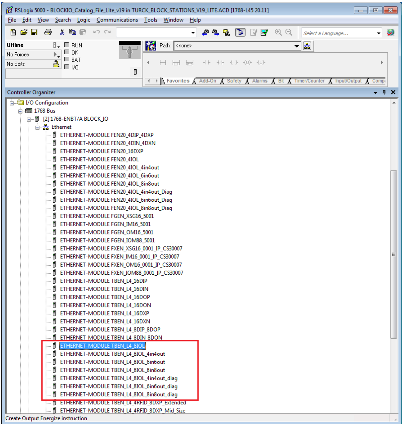
Abb. 56: RSLogix – Geräteeintrag aus Catalog-Datei kopieren
