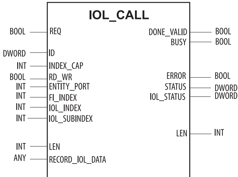
Abb. 38: IOL_CALL gemäß IO-Link-Spezifikation
