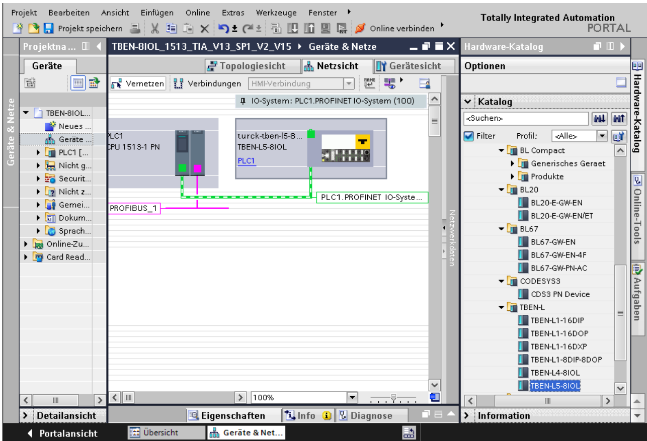
Abb. 40: Gerät mit der Steuerung verbinden
