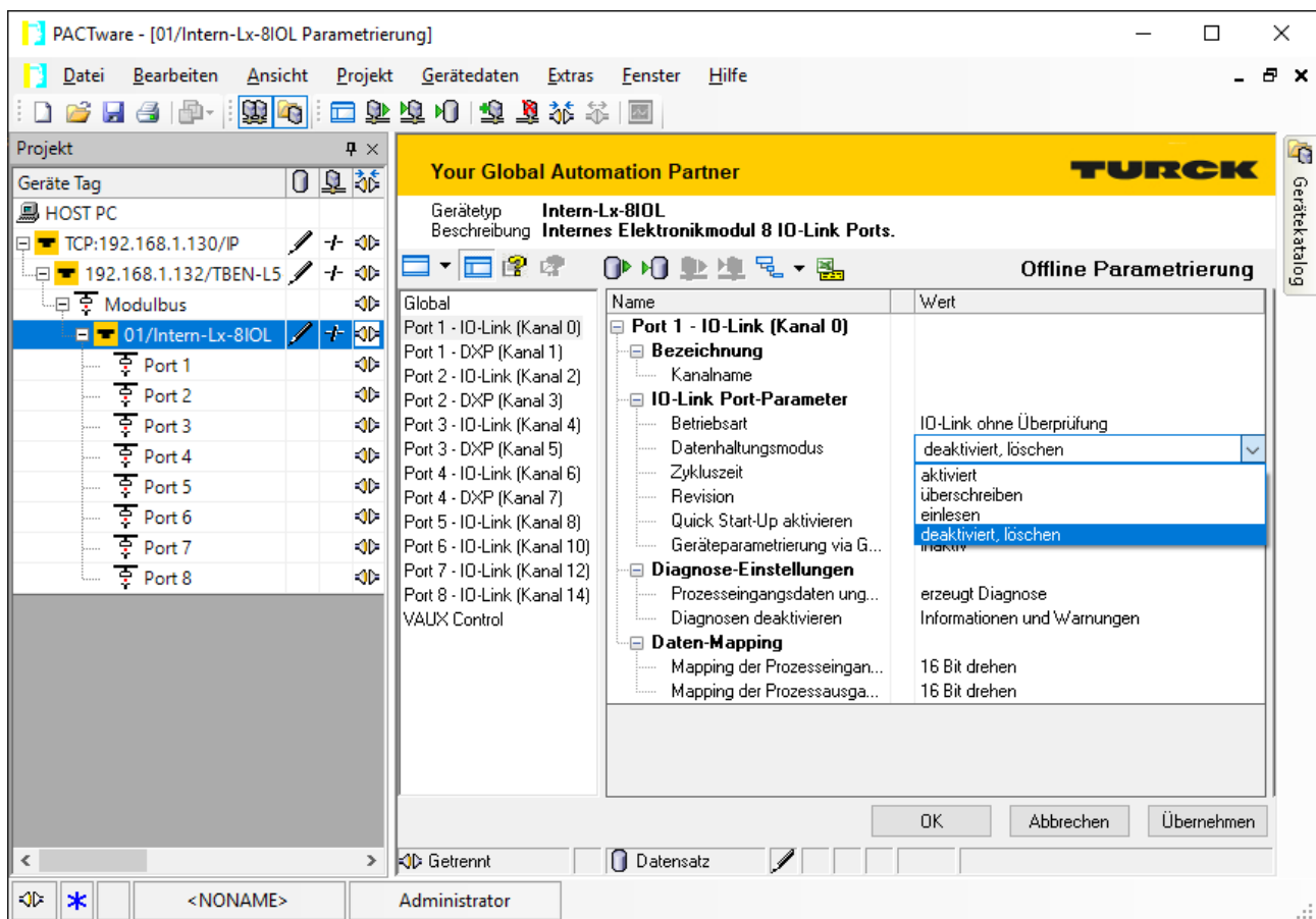
Abb. 32: Beispiel: Datenhaltungsmodus über DTM deaktivieren bzw. löschen
