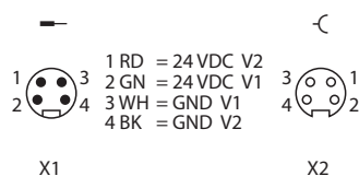
Abb. 18: TBEN-L4... – Pinbelegung Versorgungsspannungsanschlüsse
