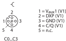
Abb. 22: Pinbelegung der IO-Link-Master-Ports, Class A, C0...C3
