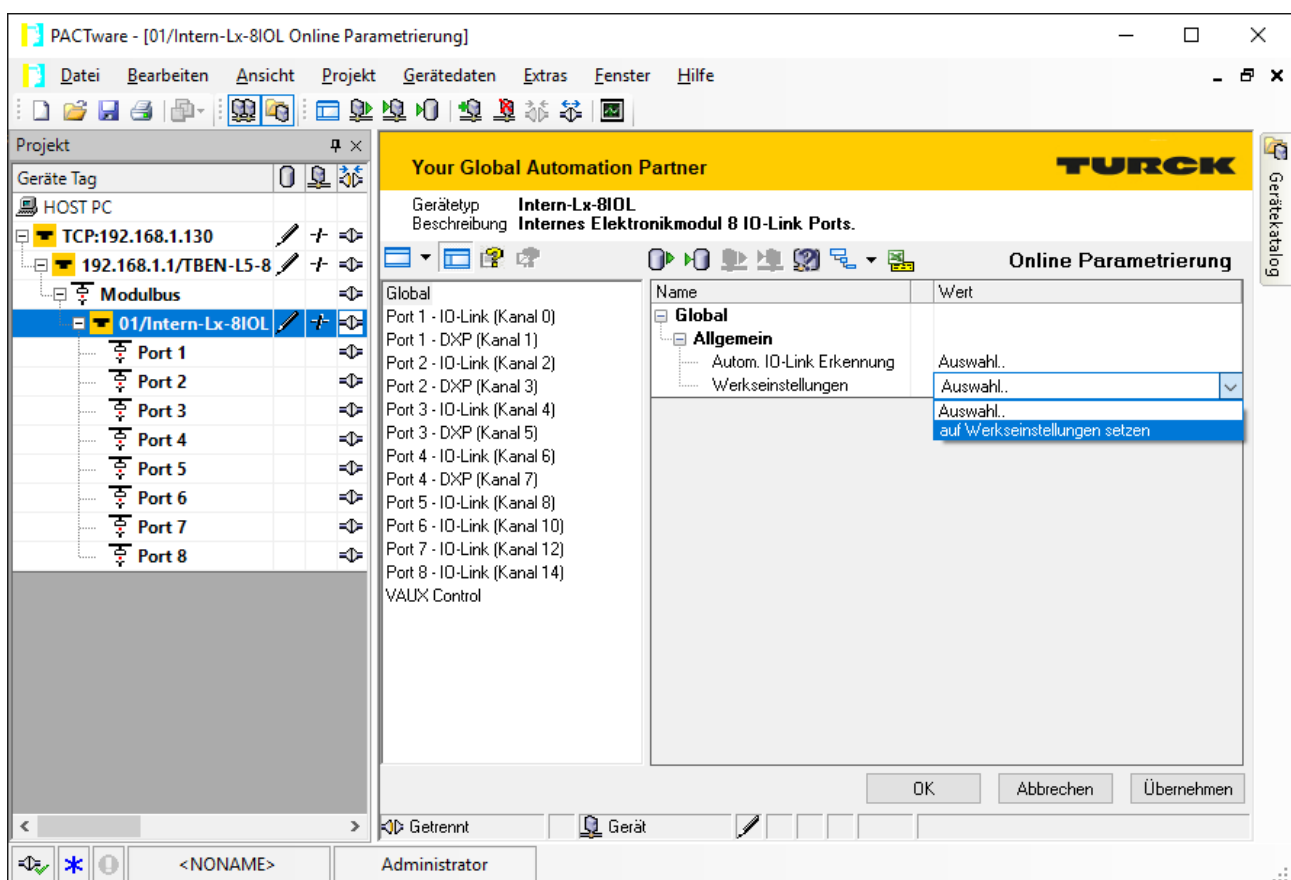
Abb. 33: Beispiel: Gerät über DTM auf Werkseinstellungen zurücksetzen
