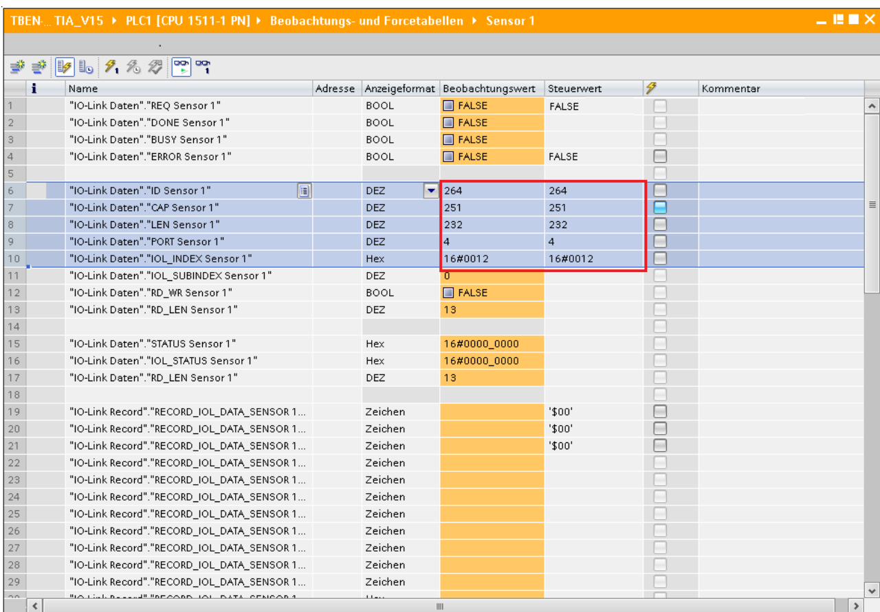
Abb. 48: IO_LINK_DEVICE – Eingangsvariablen für Lesezugriff
