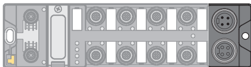
Abb. 16: TBEN-L4... – 7/8"-Steckverbinder zum Anschluss an die Versorgungsspannung
