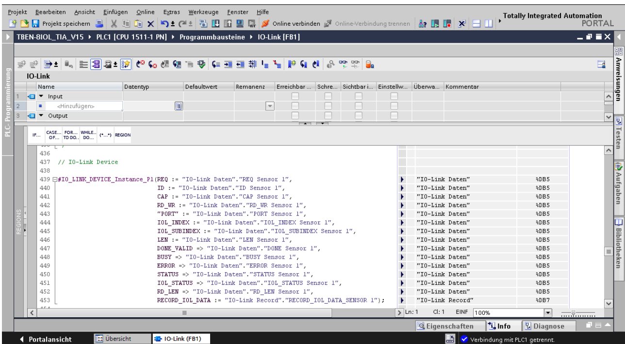
Abb. 46: Beispielaufwurf Siemens-Funktionsbaustein „IO_LINK_DEVICE“
