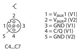
Abb. 24: Pinbelegung der IO-Link-Master-Ports, Class B, C4...C7
