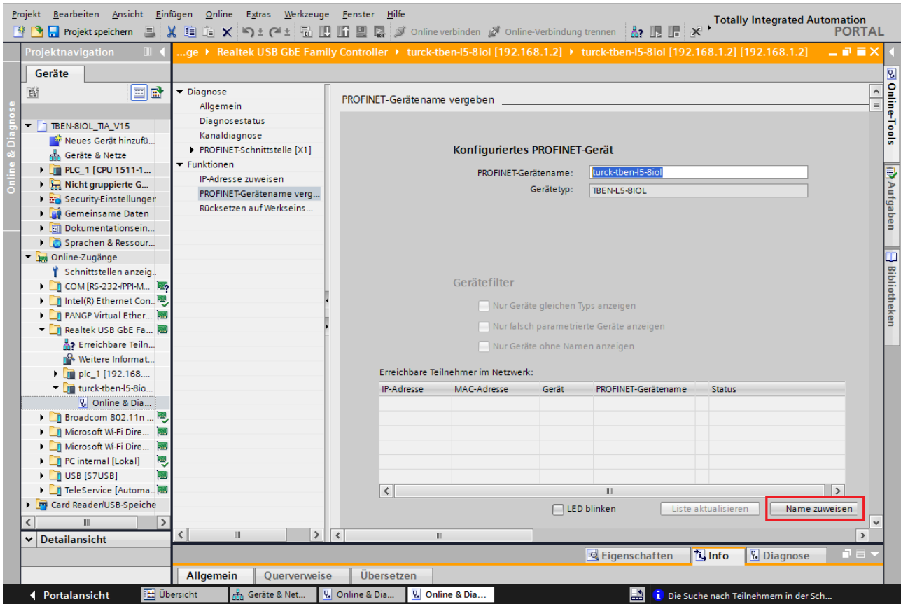
Abb. 41: PROFINET-Gerätenamen zuweisen
