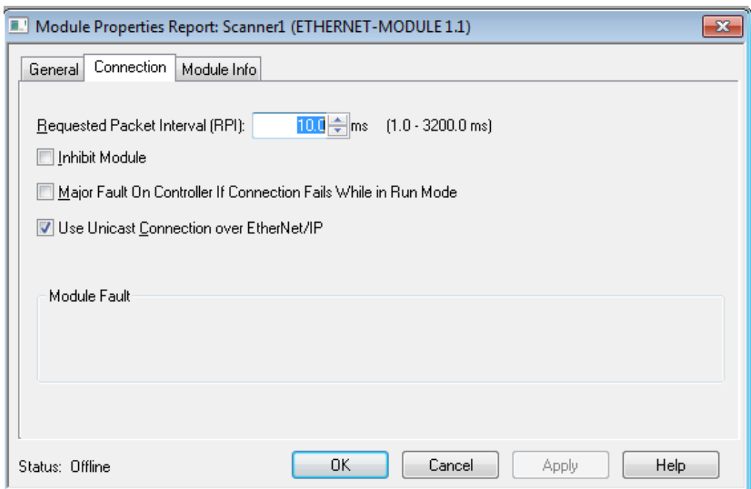
Abb. 59: Verbindung einstellen
