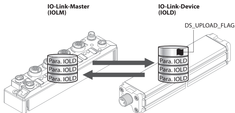
Abb. 64: Datenhaltungsmodus – generelles Prinzip, Para. IOLD = Parameter des IO-Link-Device
