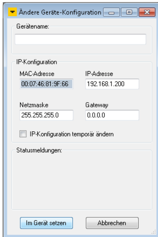
Abb. 29: Turck Service Tool – Geräte-Konfiguration ändern
